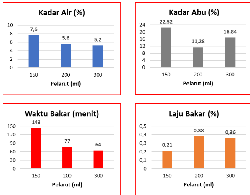
Gambar 1 Hasil Analisa Kadar Air, Waktu Bakar, Kadar Abu dan Laju Bakar (Perekat 50 gr dan Arang 100 gr)
